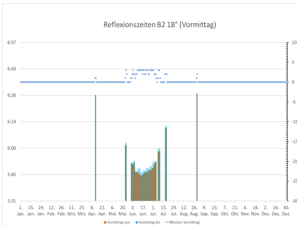
Abbildung 6: Reflexionszeiten und Dauer am Vormittag zu Punkt B2, 18° Modulneigung
