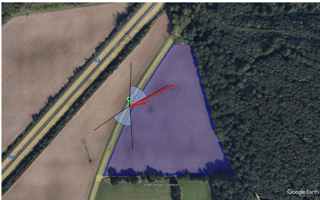
Abbildung 11: Vergleich Sichtfeld Fahrzeugführer zu Punkt B3, 18° mit Grenzvektoren in Richtung Module
