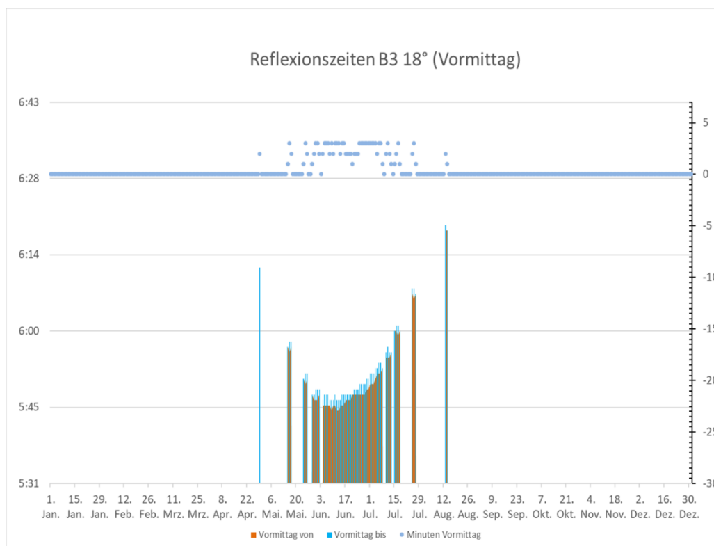
Abbildung 7: Reflexionszeiten und Dauer am Vormittag zu Punkt B3, 18° Modulneigung
