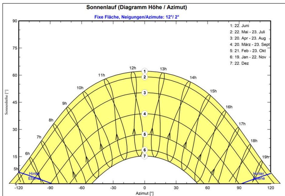
Abbildung 5: Horizontdarstellung des Sonnenlaufs
